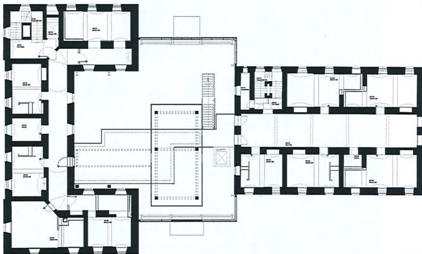
Grundriss 1. Obergeschoss • First floor plan
